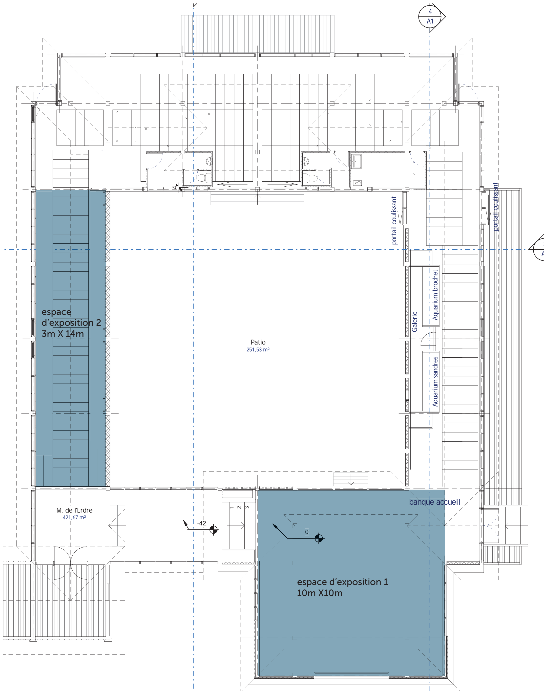
Plan de la Maison de l'Erdre Jardin japonais de l'île de Versailles Nantes 1/100 format A3
