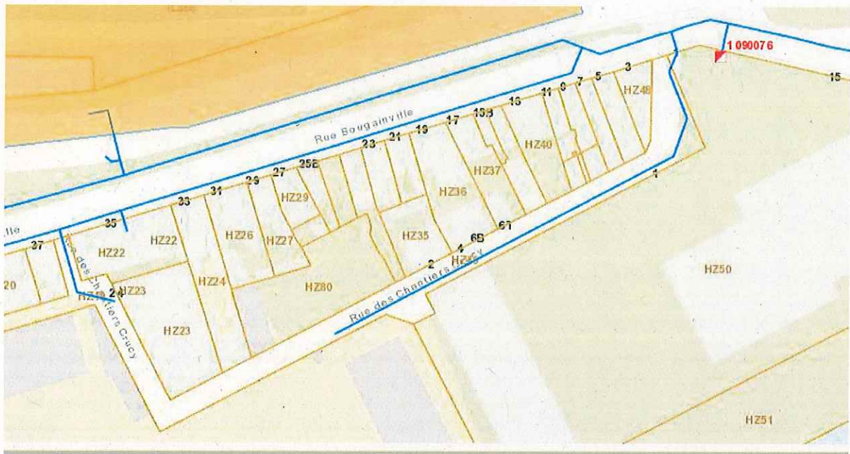
Représentation schématique du réseau d'eau potable – source : Nantes Métropole
