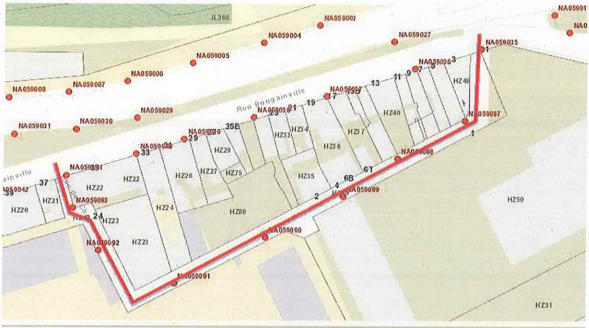
Représentation schématique de l'emplacement des point lumineux – source : Nantes Métropole
